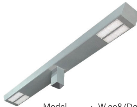
Model : W 008 (Double Arm) Dimension : L 2000 / W 200 / H 375 Power : 4 x 30w 4x60w
